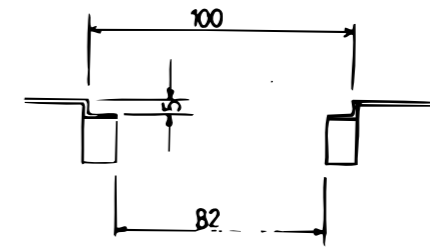
視 A-A (寸法 1/2)
